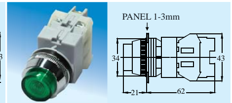
NIEPBSE-30L
