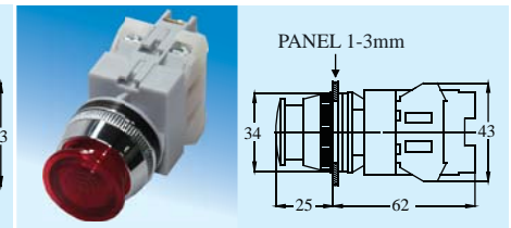
NIEPBE-30L
