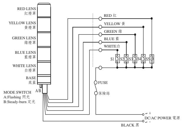
LTM/LTGM WIRING DIAGRAM 配線圖 Flashing Or Steady Mode 閃光或定光模式
